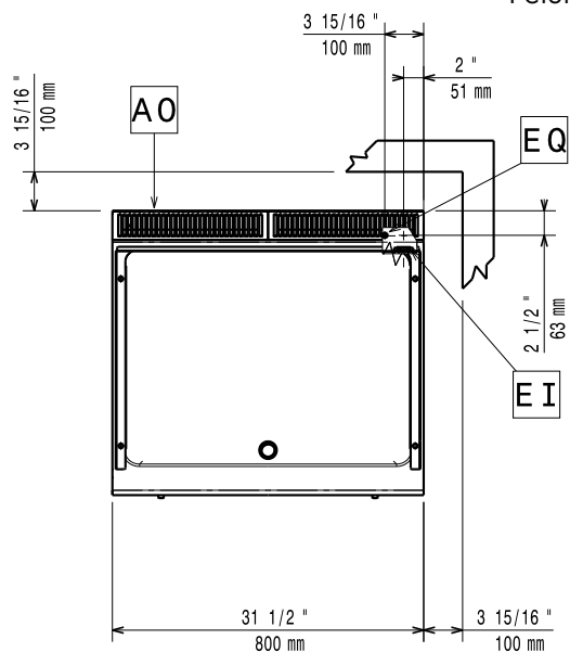
Felülnézet
